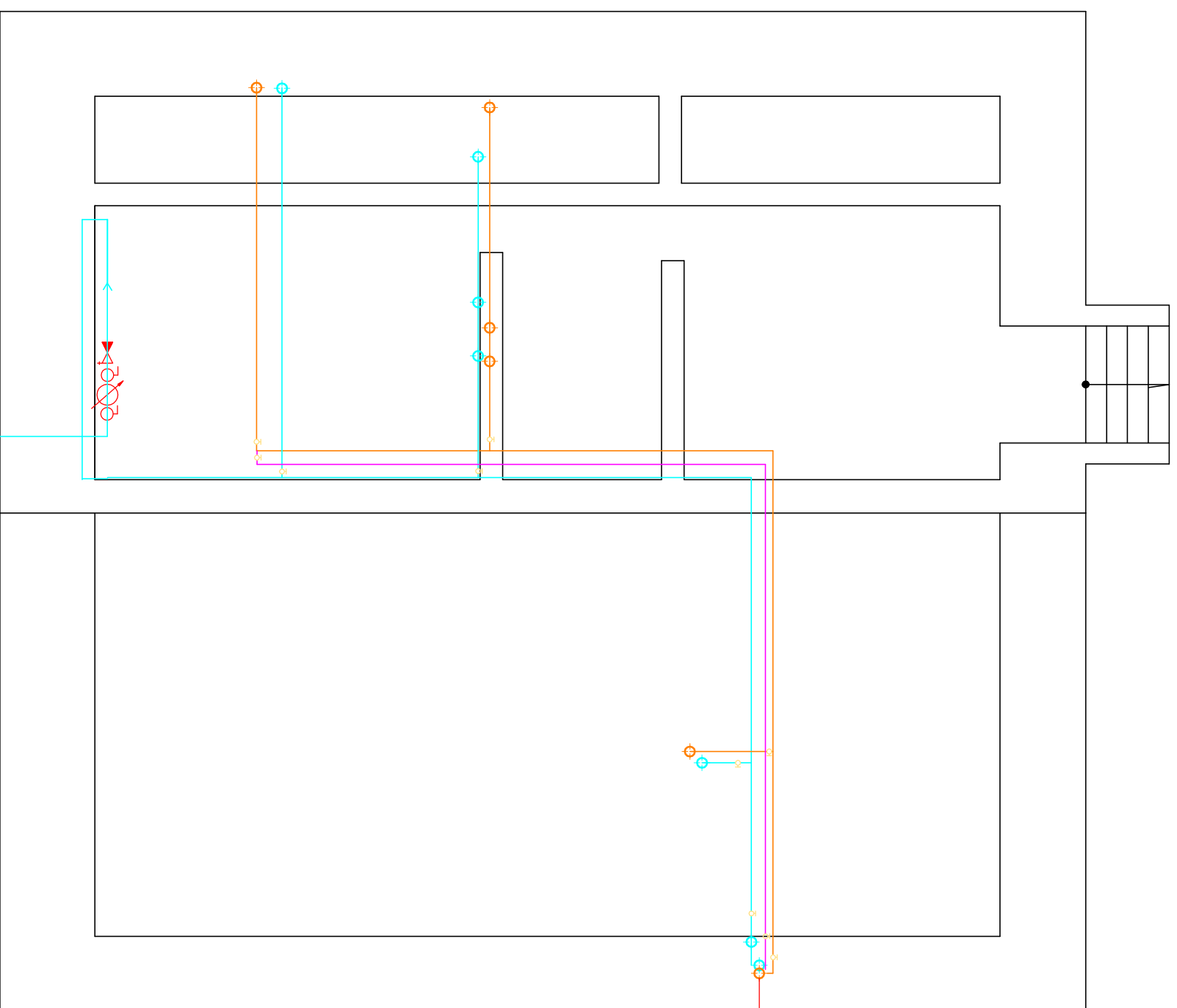
RZUT PIWNICY 1:100
