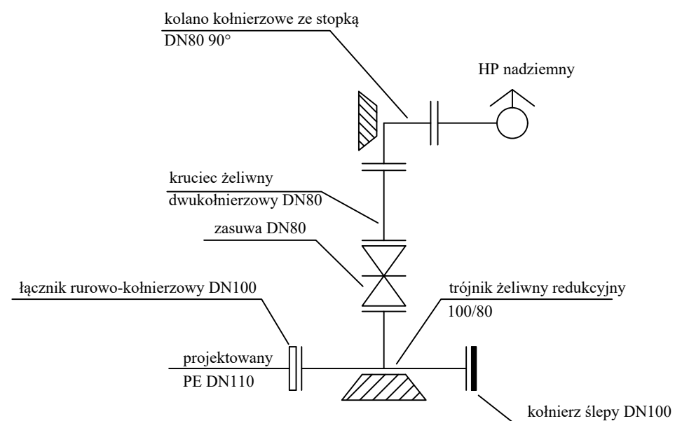
Hydrant HP2
