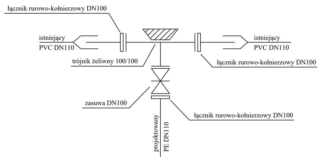
Węzeł "A"
